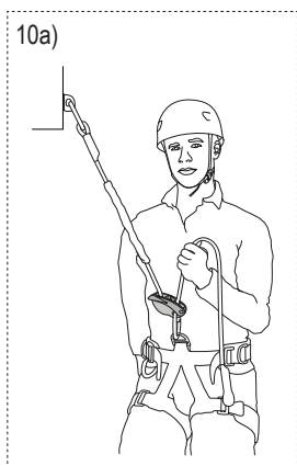
Abb. 10 Nutzung als Positionierungssystem
