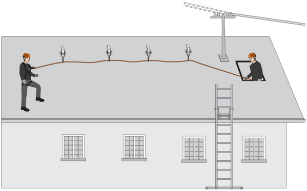
Abb. 6 Anschlageneinrichtung: temporäre Befestigung an einer Struktur
