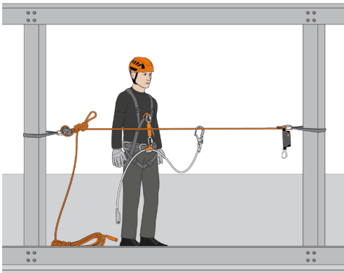
Abb. 7 horizontale Absturzsicherung (max. 2 Personen)
