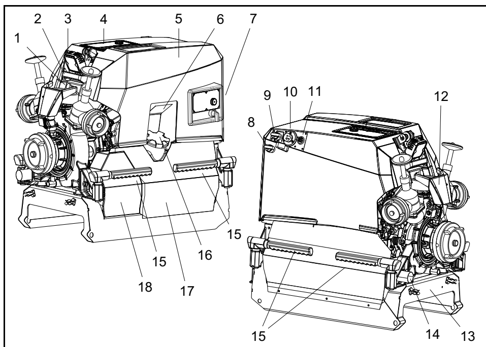
Bauteile Tragkraftspritze
