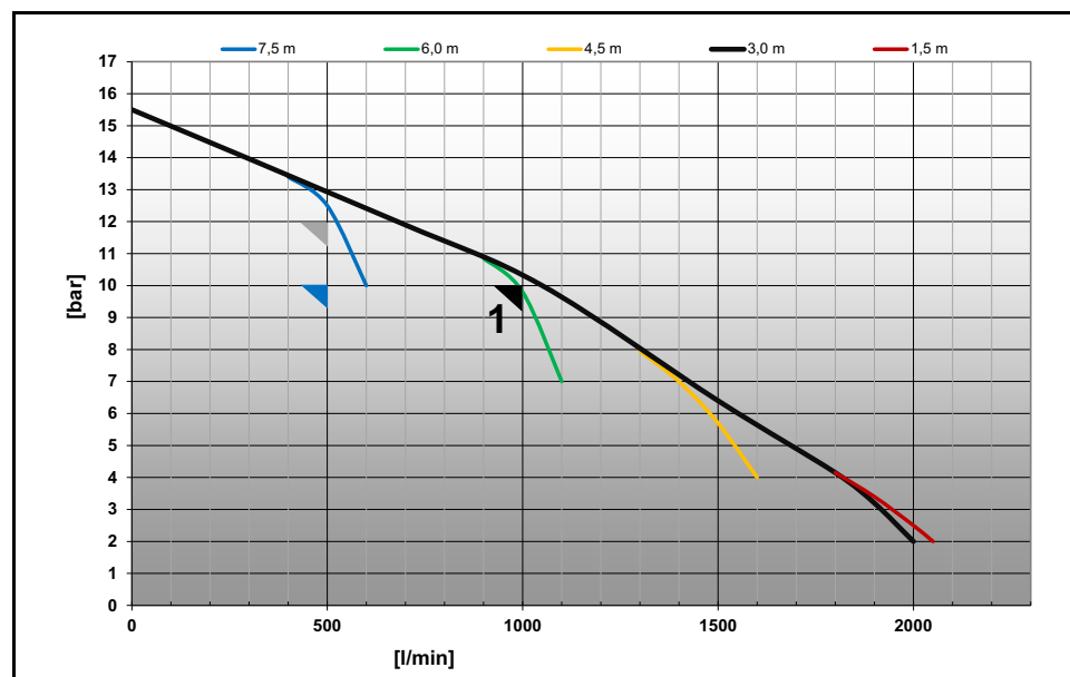
Leistungsdiagramm-Förderleistung
