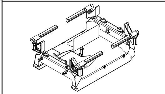
Traggestell
